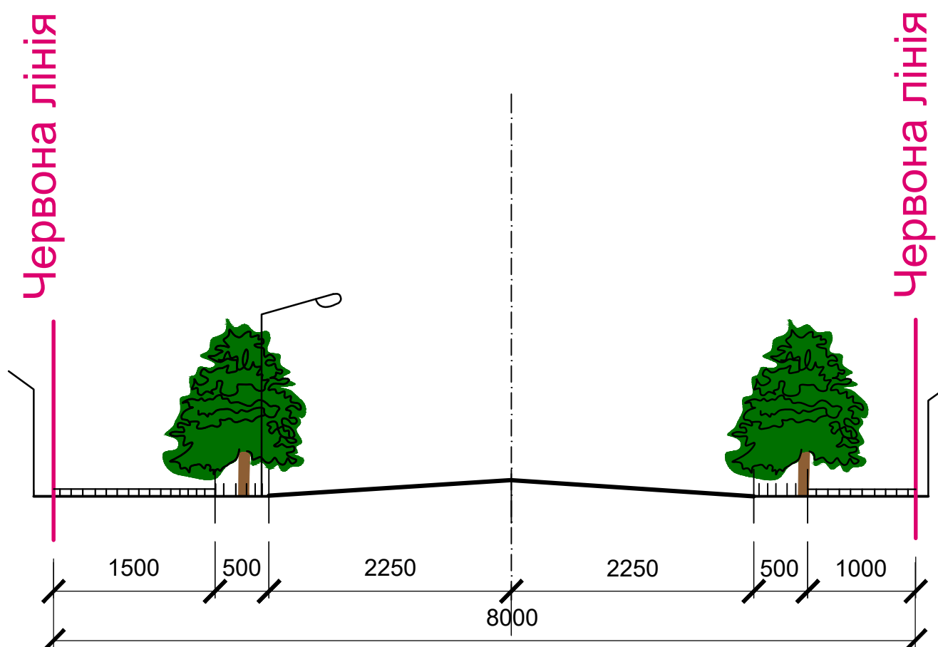
Поперечний профіль вулиці Привокзальна 1-1. М 1:50
