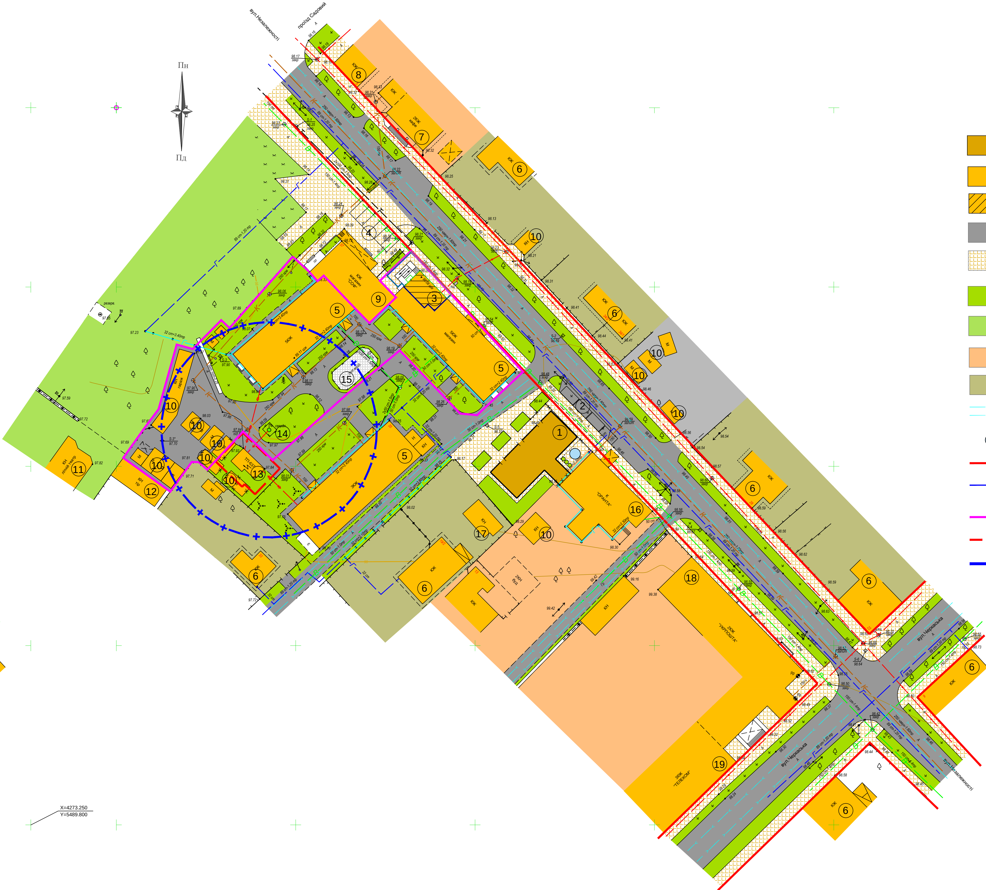
ПРОЕКТНИЙ ПЛАН, СХЕМА ПЛАНУВАЛЬНИХ ОБМЕЖЕНЬ, ПЛАН ЧЕРВОНИХ ЛІНІЙ, СХЕМА ОРГАНІЗАЦІЇ РУХУ ТРАНСПОРТУ ТА ПІШОХОДІВ. М 1:500.
