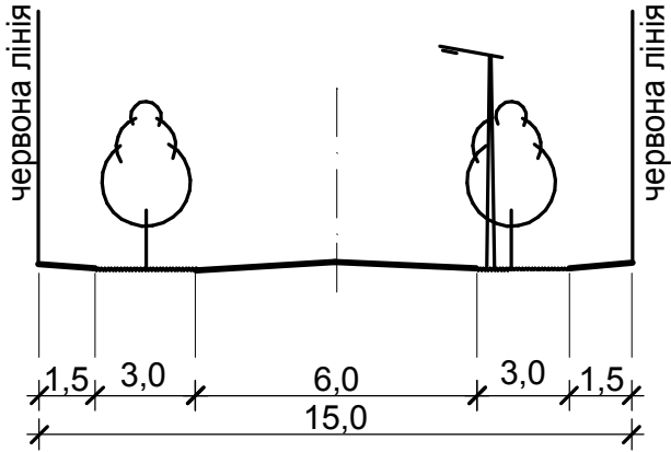
ПРОФІЛЬ ПРОВУЛКУ
