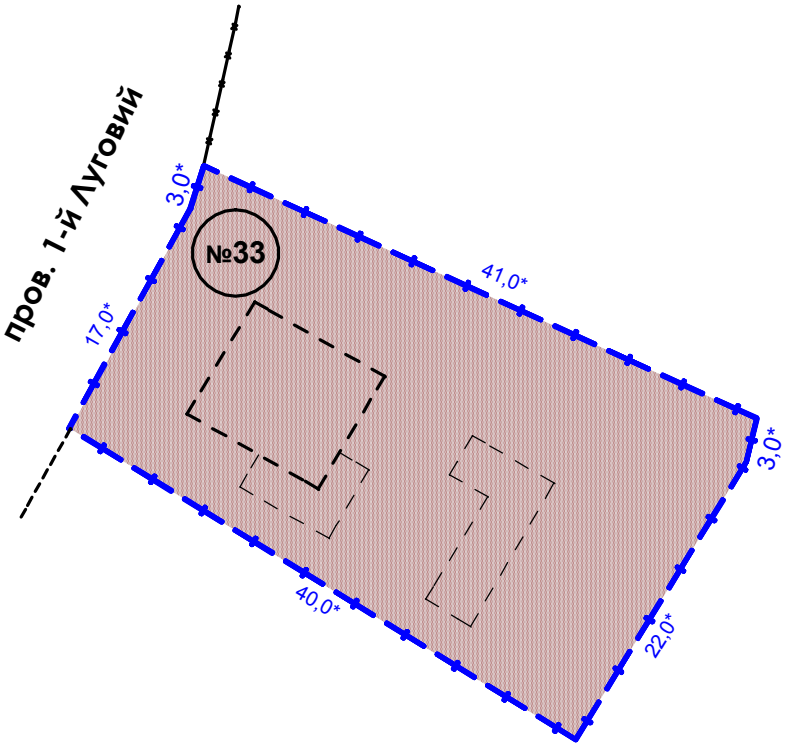
ПЛАН ДІЛЯНКИ
